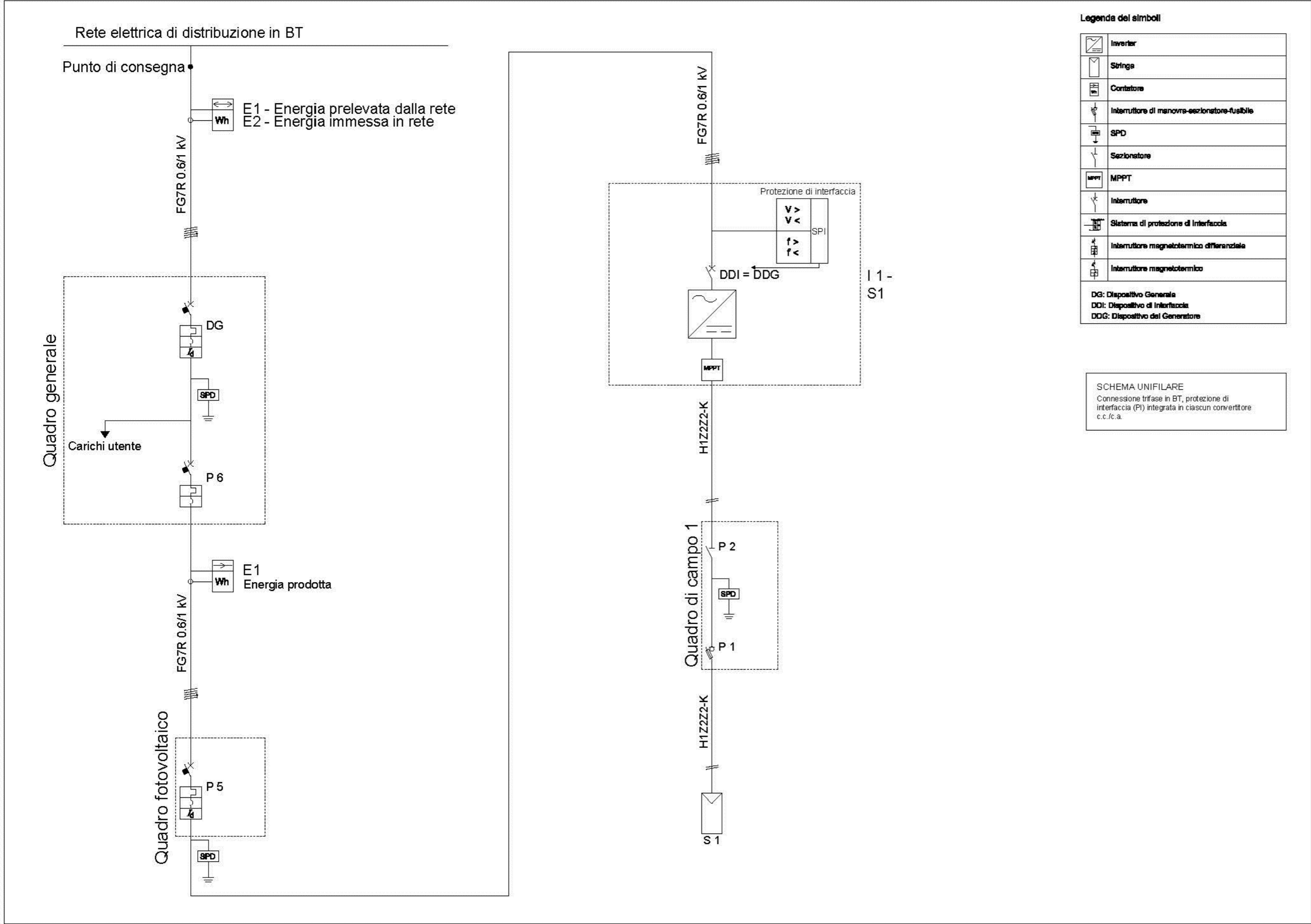
SCHEMA TIPICO IMPIANTO FOTOVOLTAICO SENZA ACCUMULO
