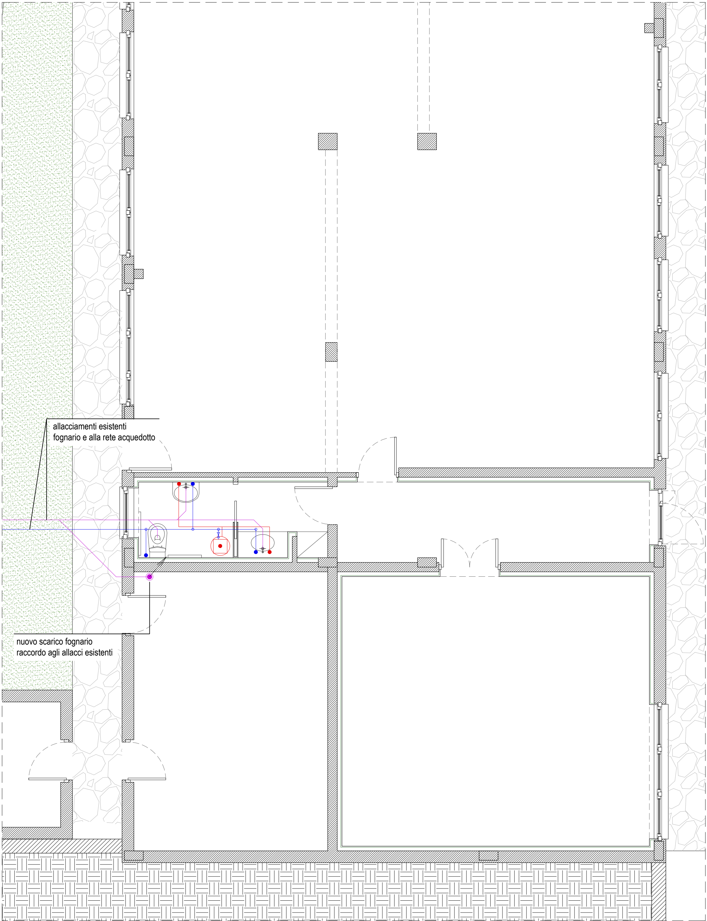
PIANTA PIANO TERRA - scala 1:50
